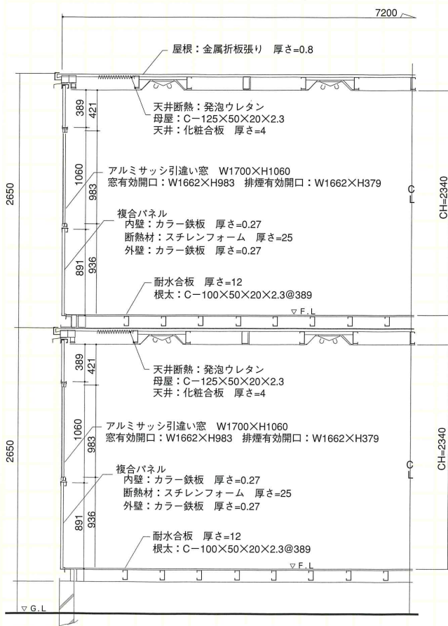
●矩計図 (CT-72DX)
