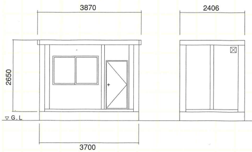
●立面図 (CT-72DX)
