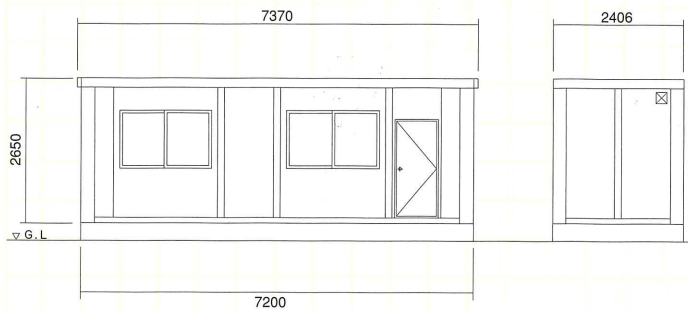
●立面図 (CT-72DX)
