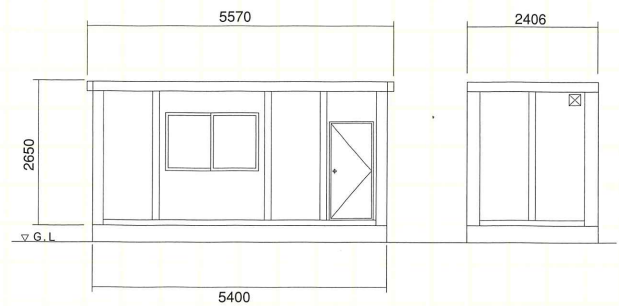
●立面図 (CT-54DX)
