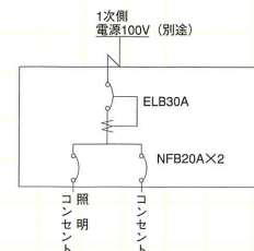
＜分電盤＞
