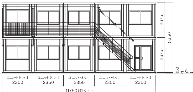
立面図
