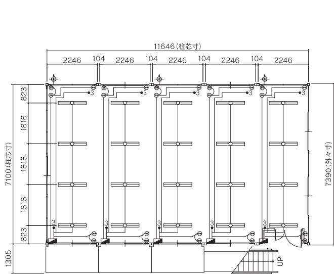
1F平面図
